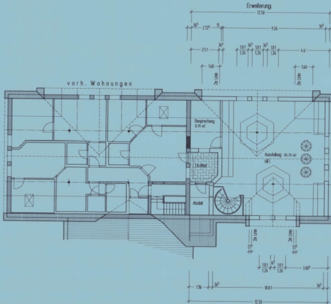
Grundriß Dachgeschoß
